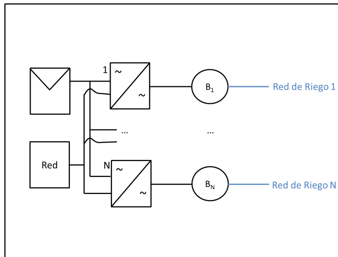
Fig 4. Sistema de riego fotovoltaico híbrido eléctricamente. La energía proviene de los generadores fotovoltaicos y de otras fuentes (grupos electrógenos o red eléctrica), y la hibridación se realiza en el circuito eléctrico.
