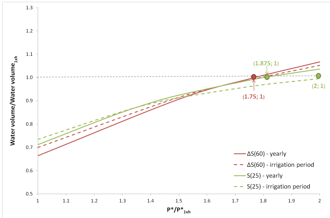
Figure 9 – Volumen de agua bombeado por un Sistema de riego fotovoltaico con estructuras ΔS(60) y S(25) normalizado por el volumen de agua bombeado por un seguidor 1xh (Water volume/Water volume 1xh ) en función de su potencia pico normalizada por la del seguidor 1xh ( P^*/P^*_{1xh} ). La línea continua representa valores anuales y la discontinua muestra los valores durante el período de riego. Los puntos con Water volume/Water volume 1xh =1 representan el sobredimensionado necesario de la potencia pico de las estructuras ΔS(60) y S(25) para igualar el servicio del seguidor 1xh.
