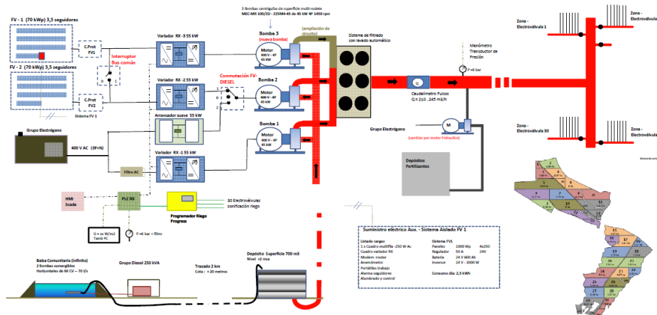
Fig. 10. Esquema de la configuración del sistema híbrido fotovoltaico-diésel de Alter do Chão. A las dos bombas del sistema se ha añadido una nueva (la más arriba en la figura) que se puede alimentar sólo desde el generador FV. Los distintos modos operación son elegidos automáticamente en función de la irradiancia que incide sobre el generador fotovoltaico.
