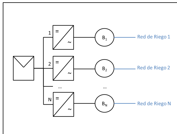
Fig 2. Sistema de riego fotovoltaico autónomo. La energía proviene exclusivamente de los generadores fotovoltaicos. La parte en negro representa la parte eléctrica, y la azul la parte hidráulica.
