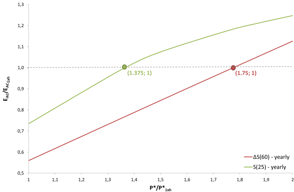
Fig. 1 – Energía anual AC producida por un Sistema fotovoltaico conecta a red con estructuras \Delta S(60) y S(25) normalizada por la energía AC producida por un seguidor 1xh ( E_{AC}/E_{AC1xh} ) en función de la potencia pico normalizada por la potencia pico del seguidor 1xh ( P^*/P^*_{1xh} ). Los dos puntos con E_{AC}/E_{AC1xh} = 1 representan el sobredimensionado necesario de la potencia pico de las estructuras \Delta S(60) y S(25) para igualar el servicio entregado por el seguidor 1xh.
